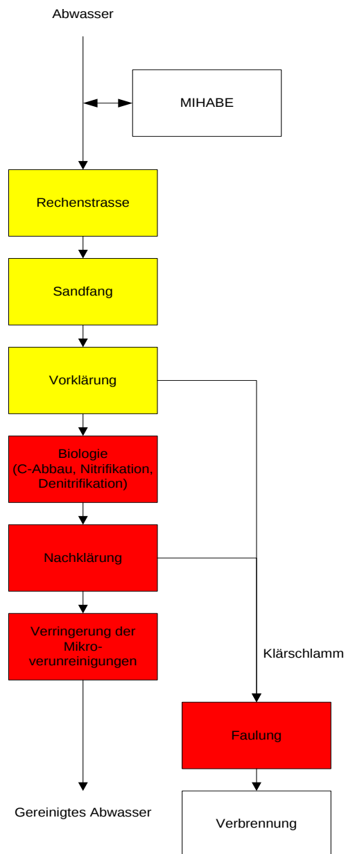
Fliessschema nach Umbau Gelb: Anlagenteile welche ertüchtigt werden Rot: Anlagen welche neu erstellt werden
