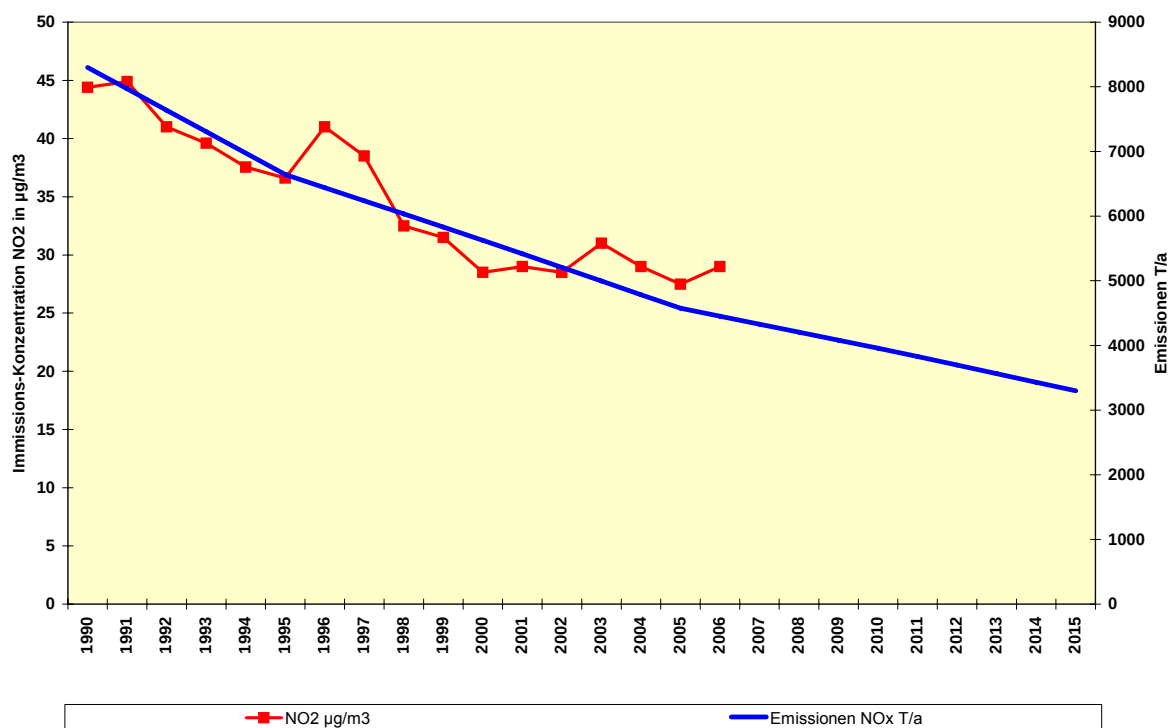
Abb. 3: Mittlere \text{NO}_2 -Immissionsbelastung in der Region Basel und Entwicklung der Emissionen 1990-2015
