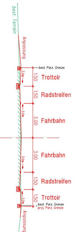
Regelquerschnitt 1:100 Baselstrasse
