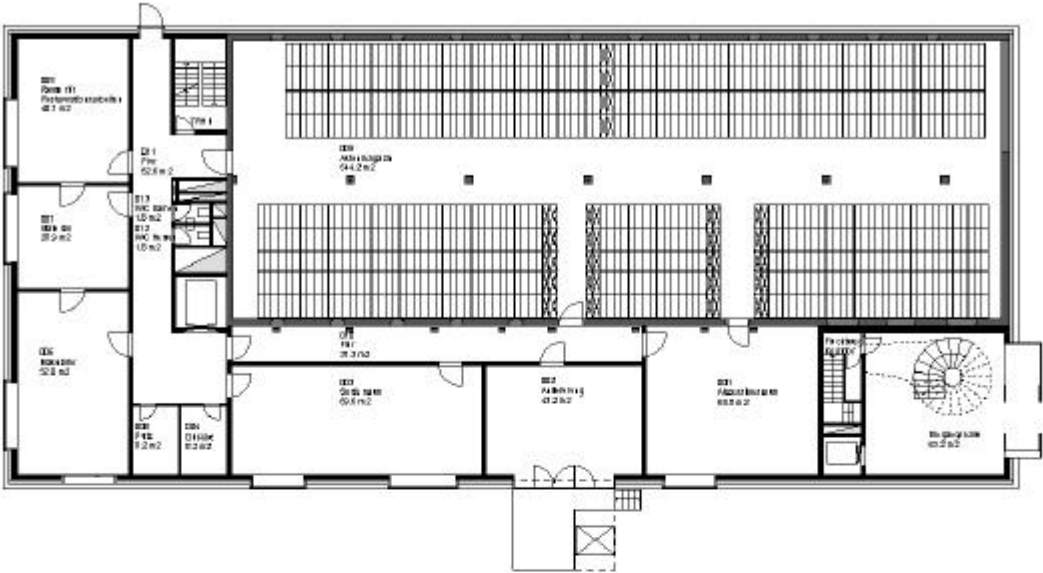
Erdgeschoss
