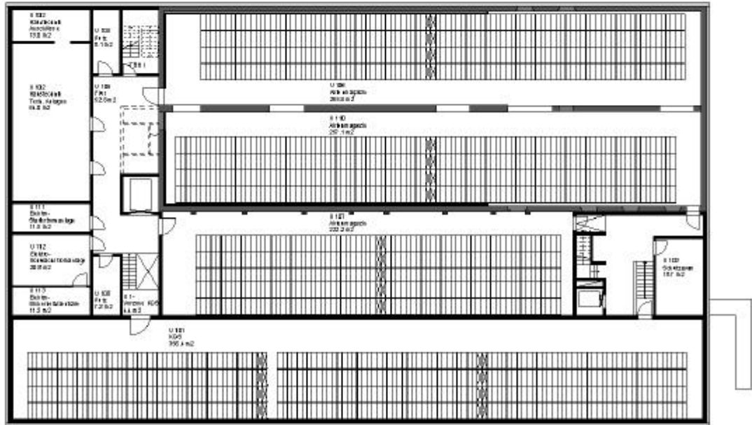
Untergeschoss
