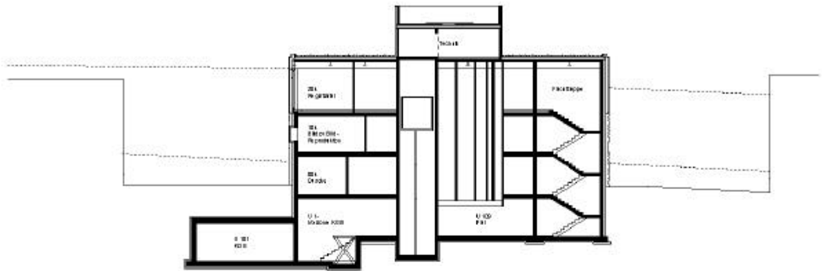
Schnitt D-D
